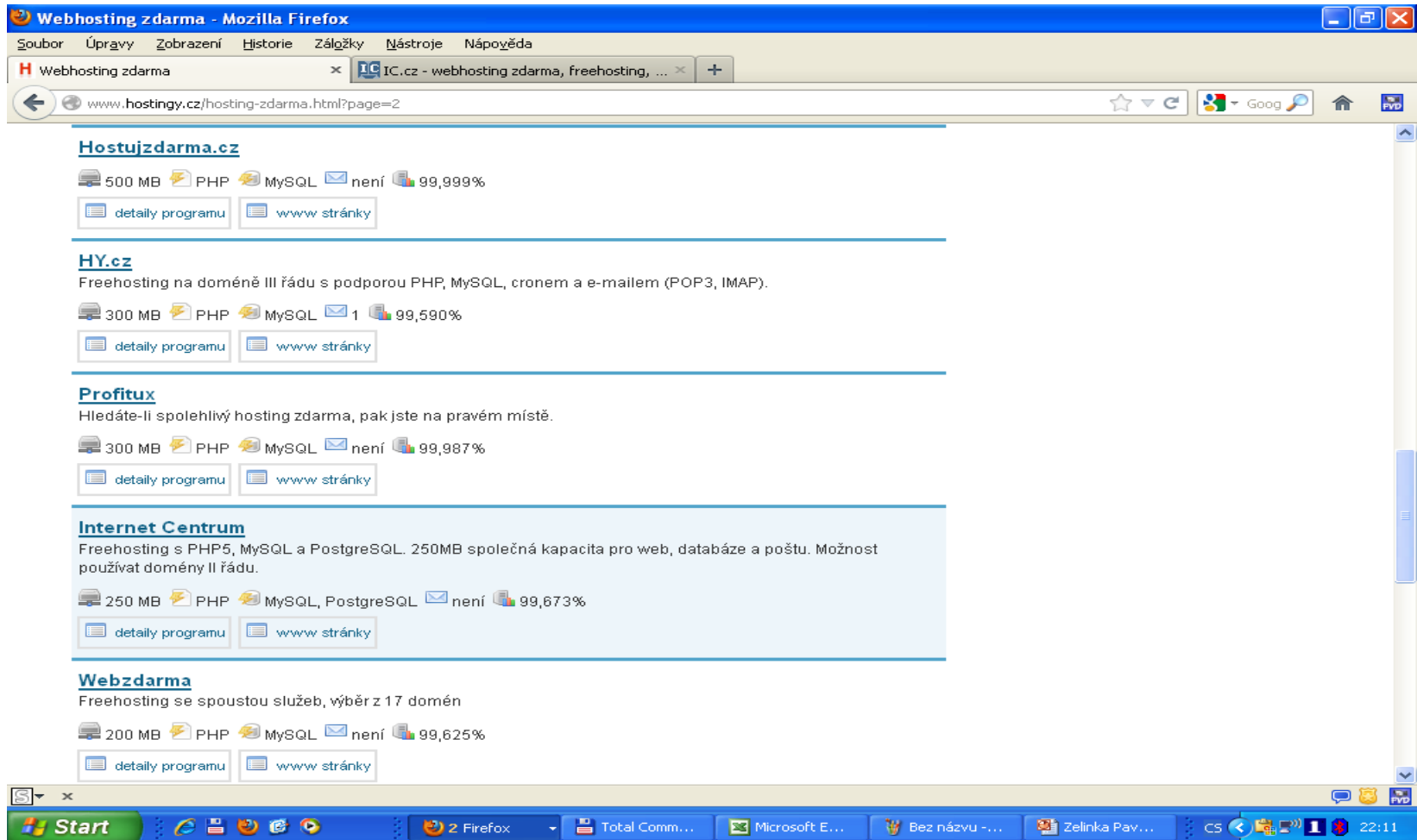
Obr. 4 Výsledky vyhledávání
